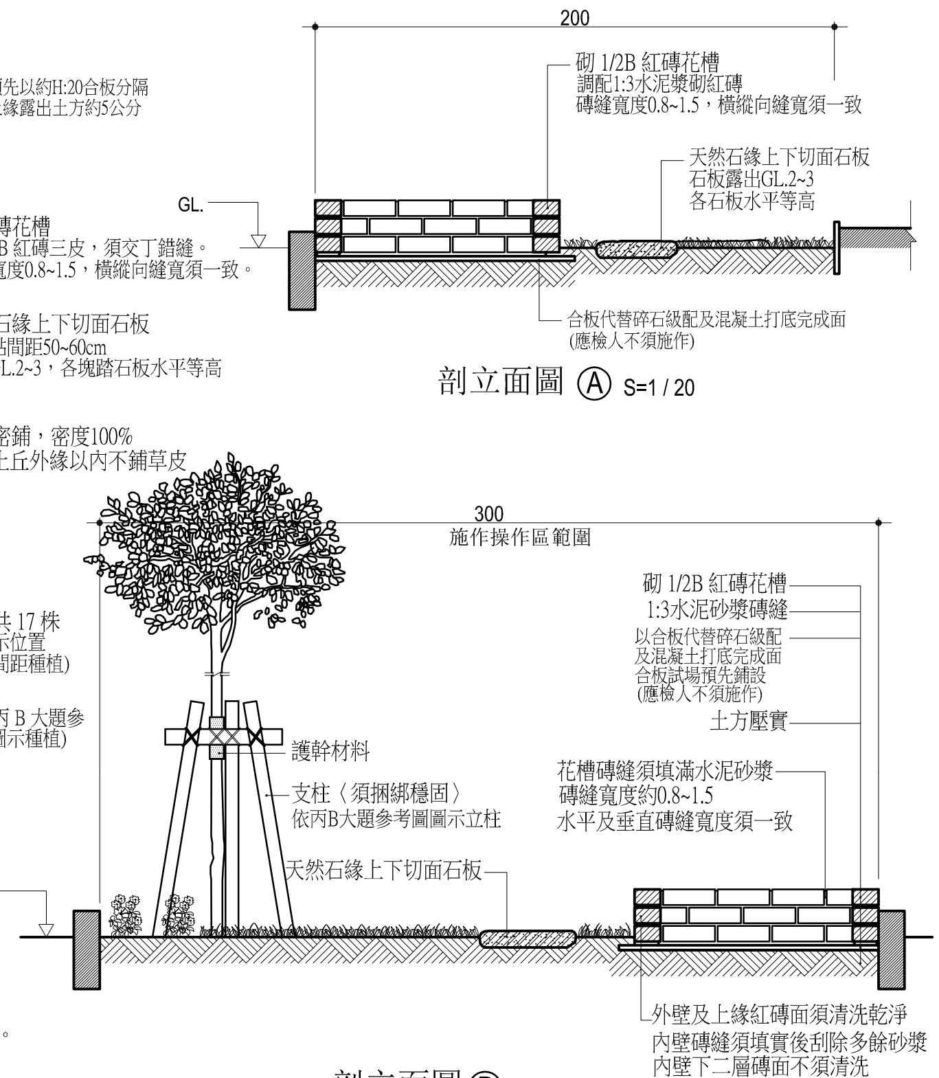
剖立面圖 (B) S=1/20
