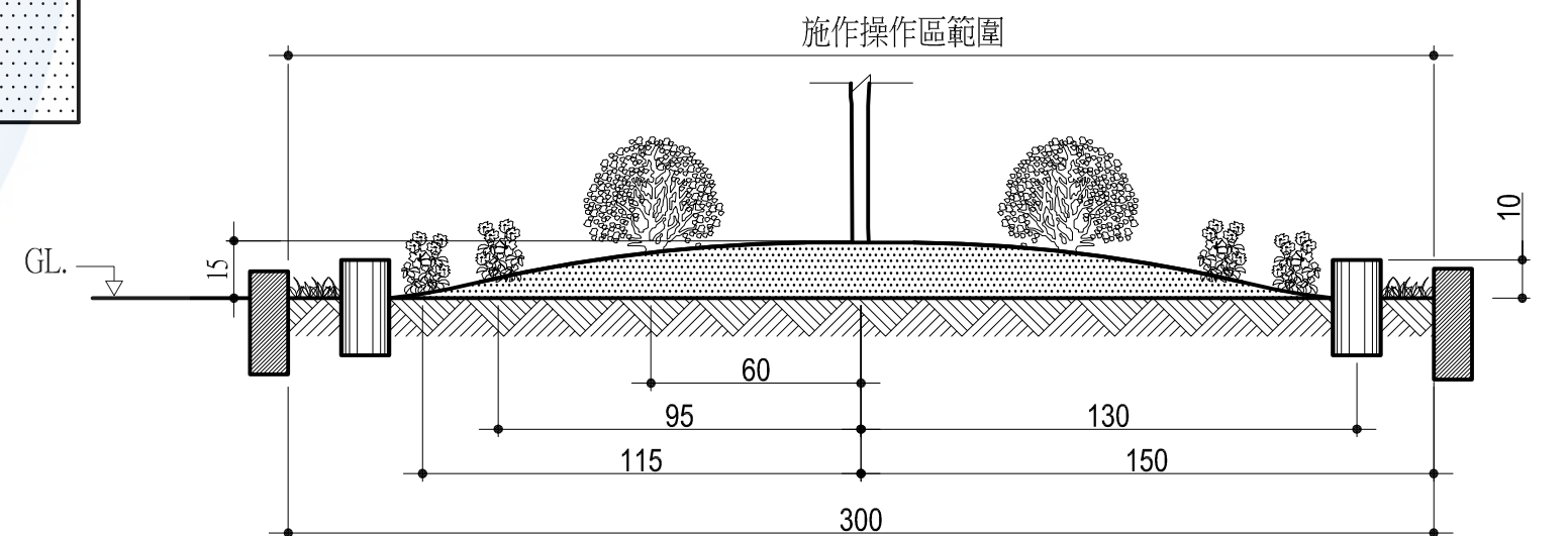
剖面圖 B S=1 / 20
