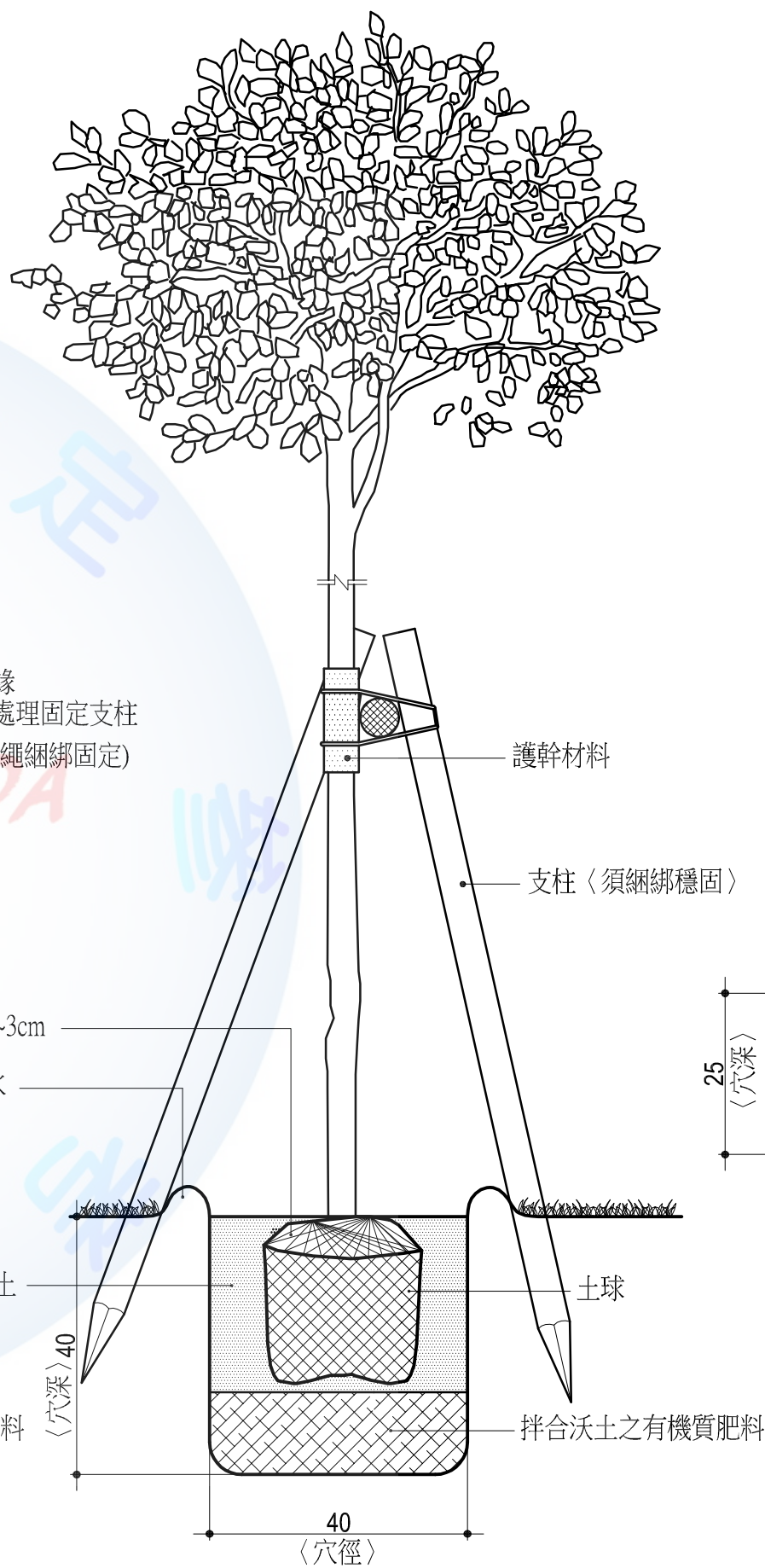
喬木栽植剖面示意圖〈側面〉S=1 / 10
