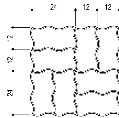
高壓水泥連鎖磚鋪設大樣示意圖 S=1/10
