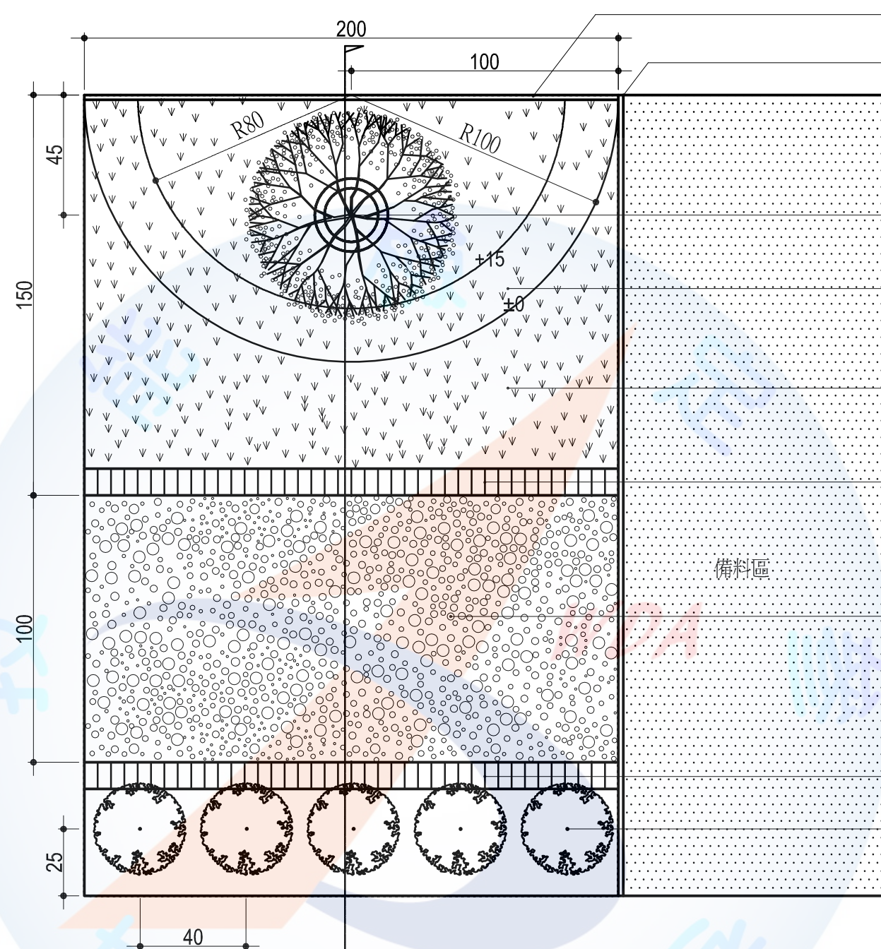
平面圖 S=1/20
