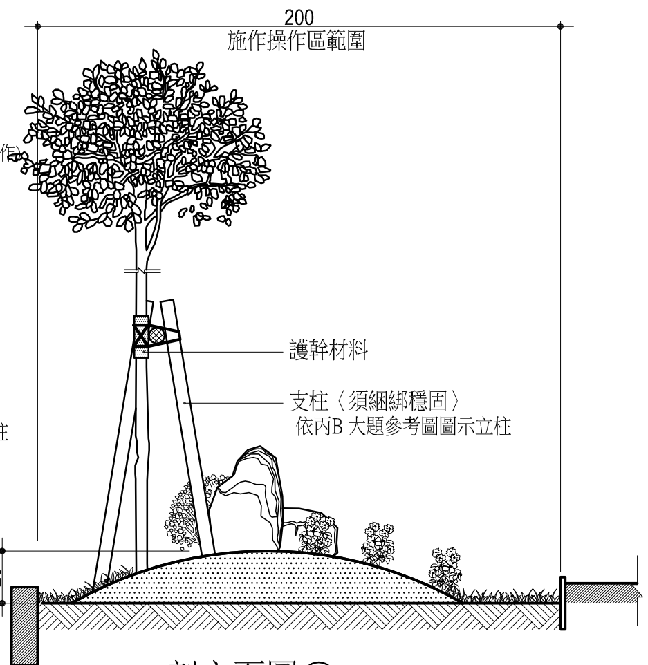
剖面圖 A S=1/20
