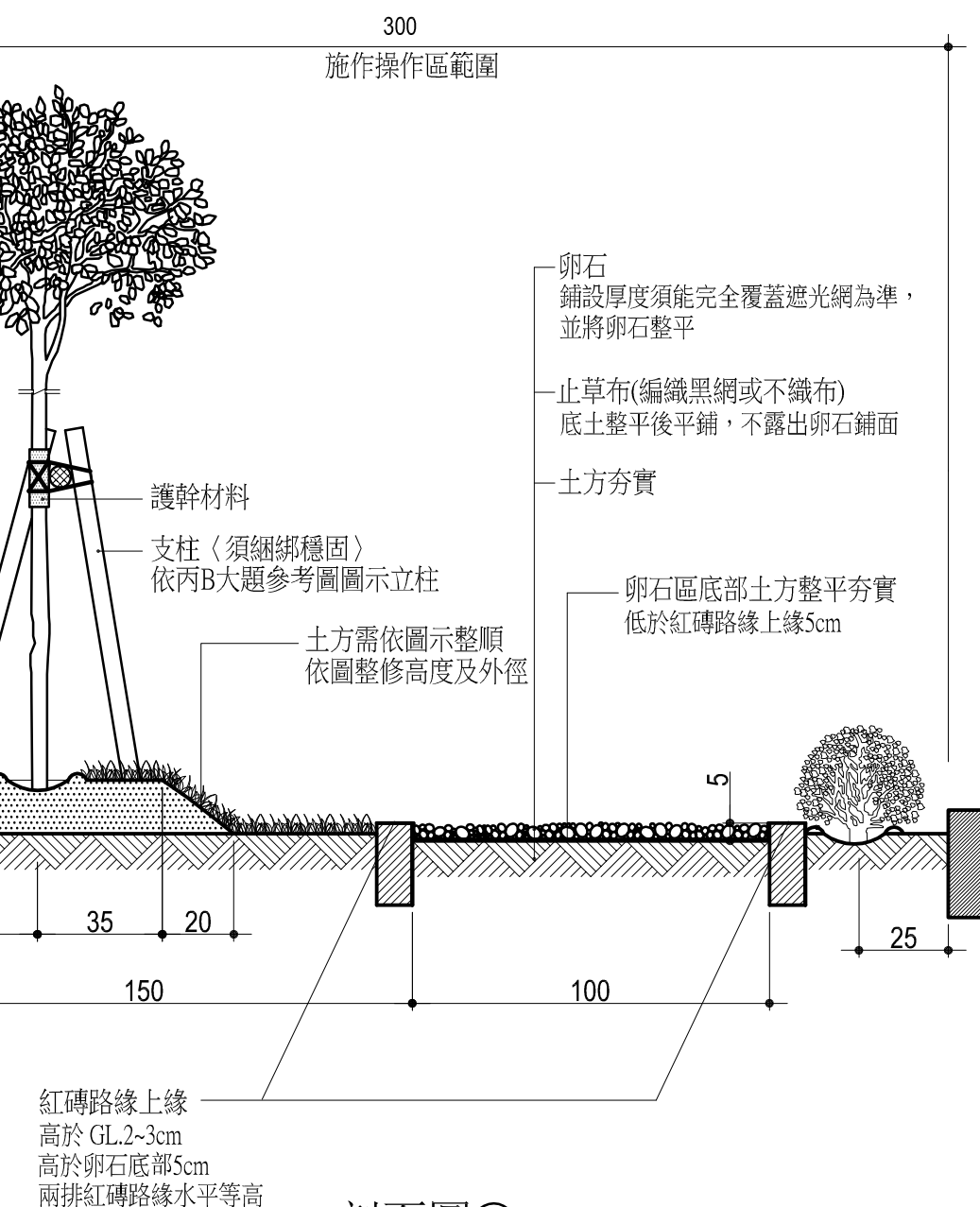
剖面圖① S=1/20
